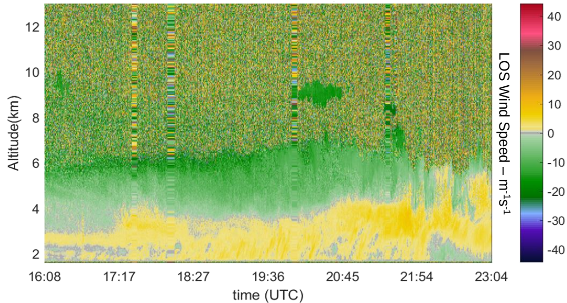
OAWL LOS Winds (m/s): 355 nm
